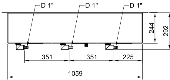
Zij aanzicht
