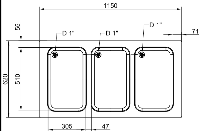
Boven aanzicht
